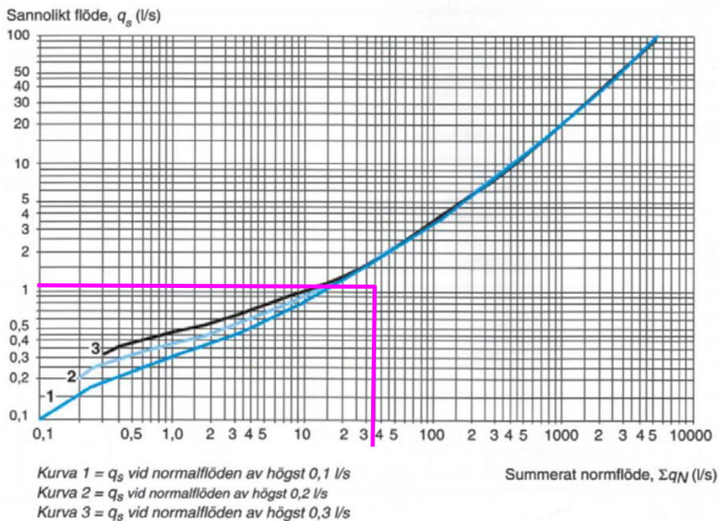
Figur 12. Dimensionerande sannolikt flöde enligt Figur 3.8 i P114.
